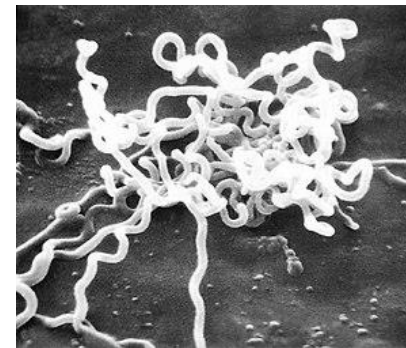
Treponema pallidum
